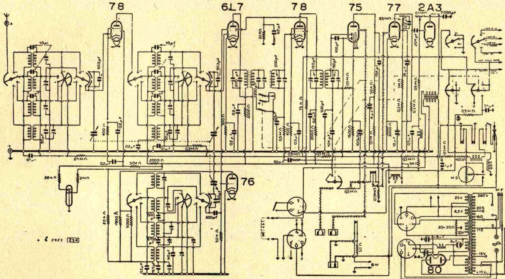
Lo schema elettrico del mod. 844/P
